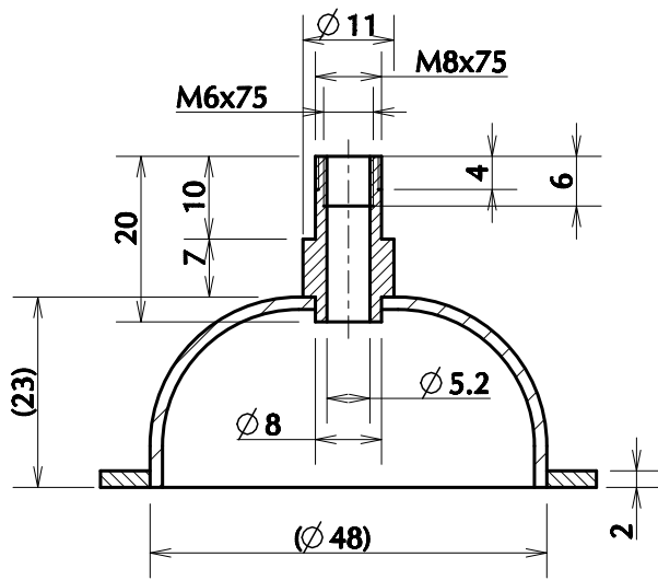
COUPE A-A
