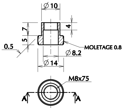
COUPE A-A
