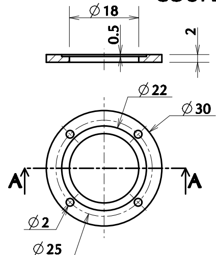
COUPE A-A
