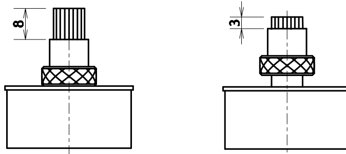
REGLAGE DE LA HAUTEUR DE MECHE
