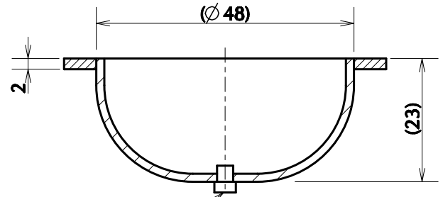
COUPE A-A
