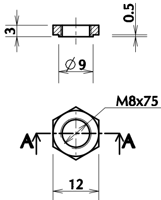
COUPE A-A
